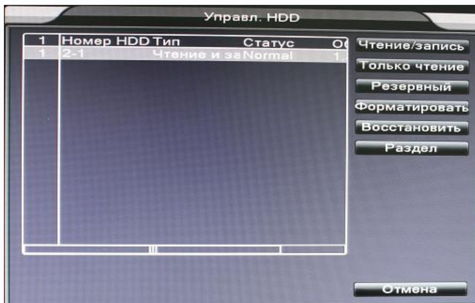
Рис. 4.32 Управление HDD
