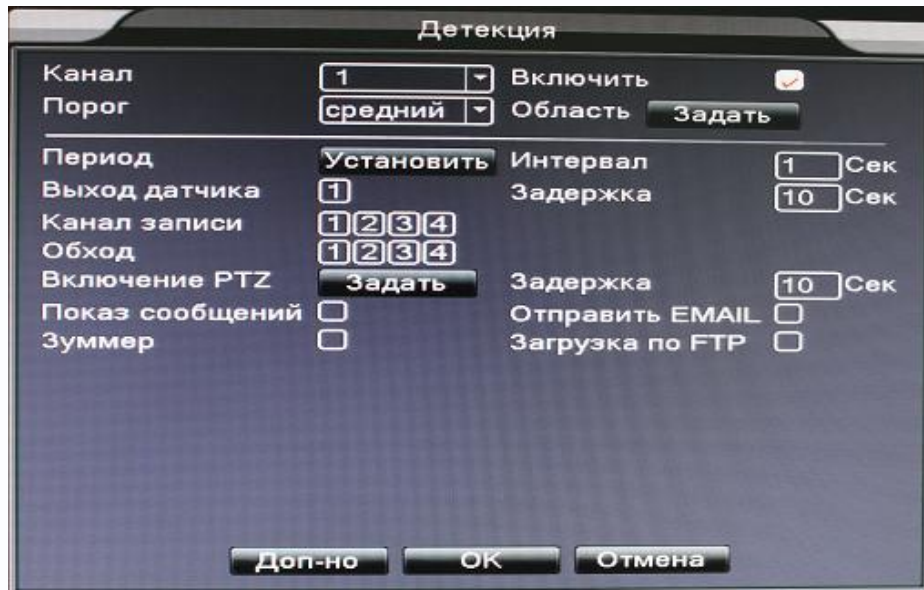
Рис. 4.4 Детектор движения
