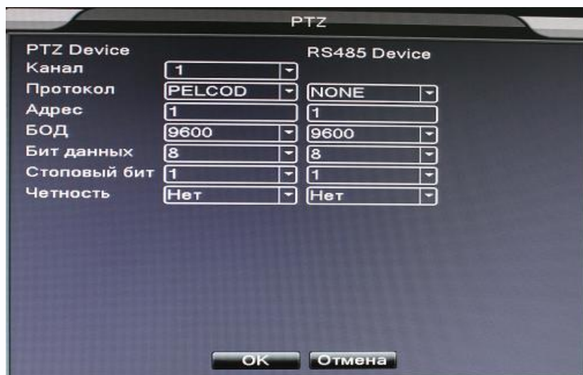
Рис. 4.29 Настройки PTZ
