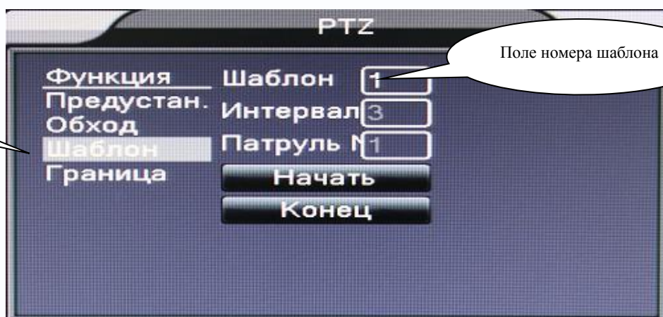
Рис. 3.14 Настройка шаблона
