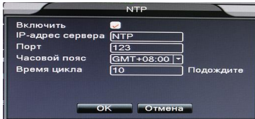
Рис. 4.20 Настройки NTP
