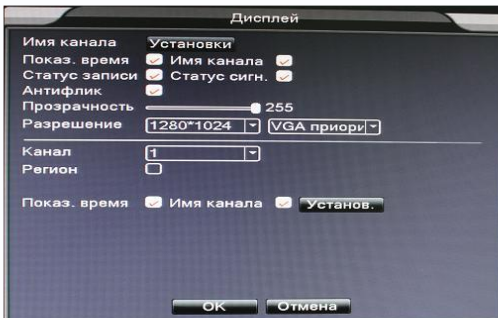
Рис. 4.28 Меню экрана
